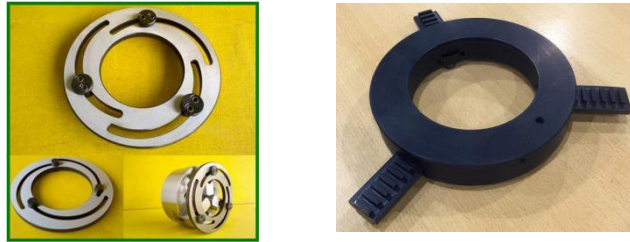
图2 软爪修调器
